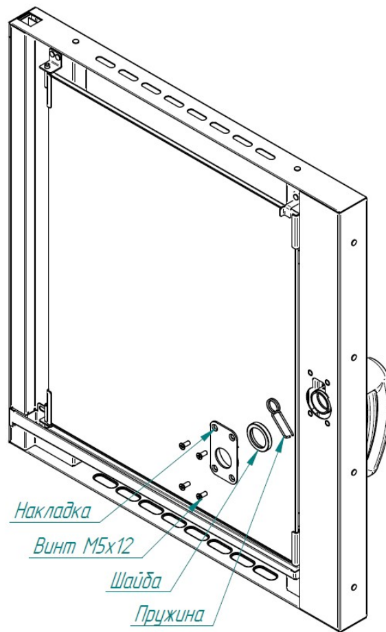
Рис.17. Ремонт замкового устройства
